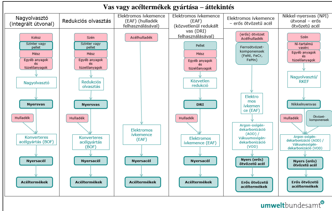
5-5. ábra: A vas- vagy acéltermékek előállításának rendszerhatárai és értéklánca
