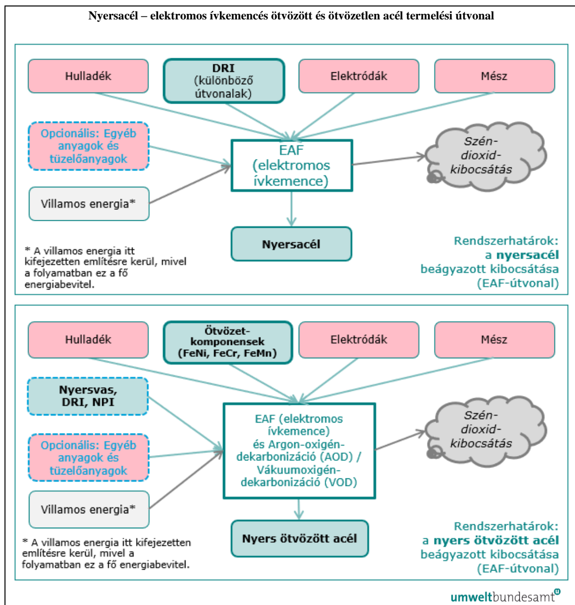
5-13. ábra: A nyersacél – elektromos ívkemencés acélgyártási termelési útvonal rendszerhatárai.
