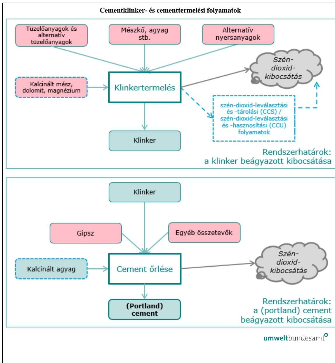
5-1. ábra: A cementklinker- és a cementtermelési folyamatok rendszerhatárai.
