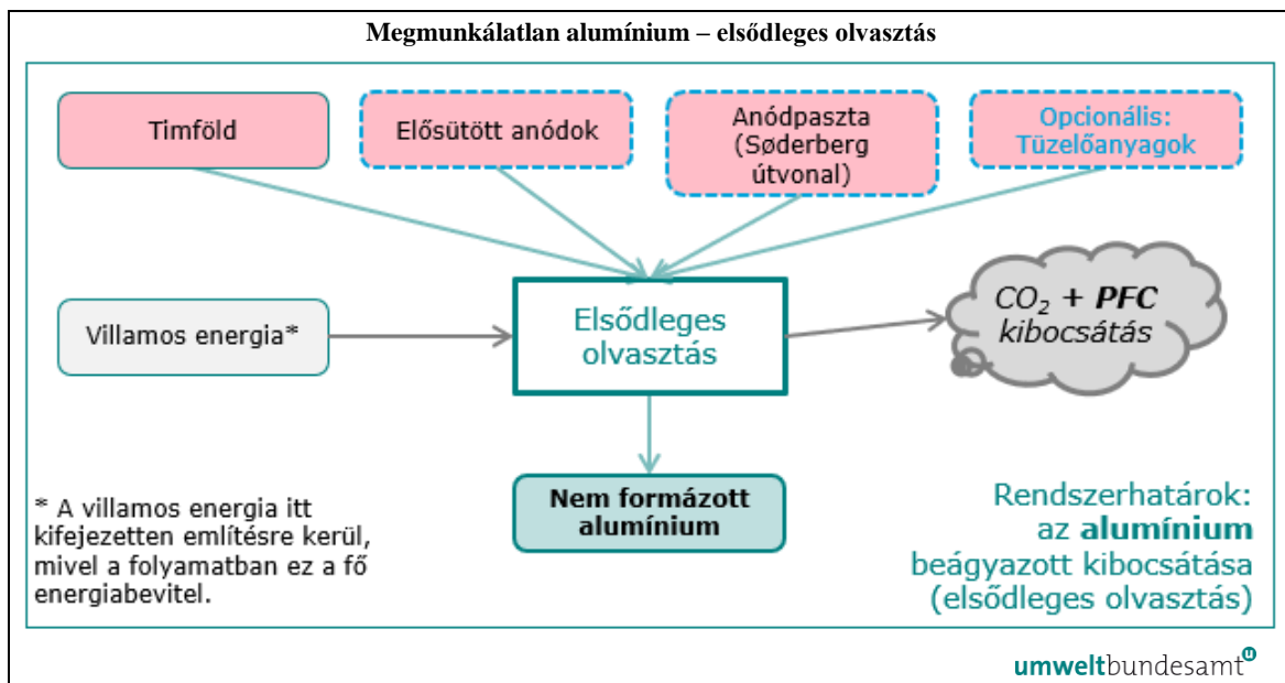
5-17. ábra: A megmunkálatlan alumínium – elsődleges olvasztás termelési útvonalának rendszerhatárai
