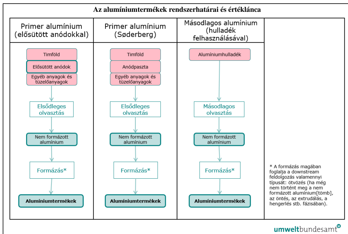
5-16. ábra: Az alumíniumtermékek rendszerhatárai és értéklánca.
